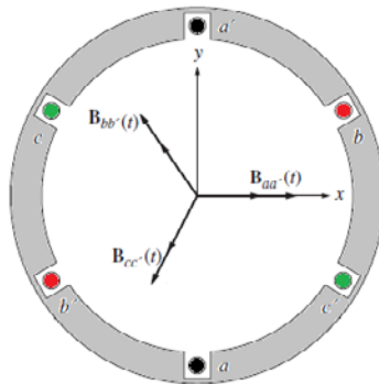
Figura 1.8 Flujos presentes en un devanado trifásico.
