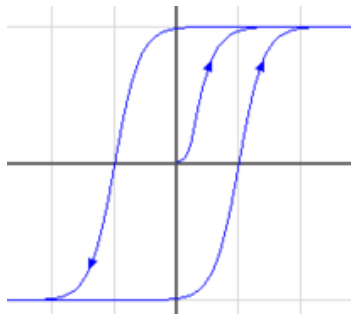
Figura 1.14 Curva de Histéresis de un material ferromagnético. [7]
